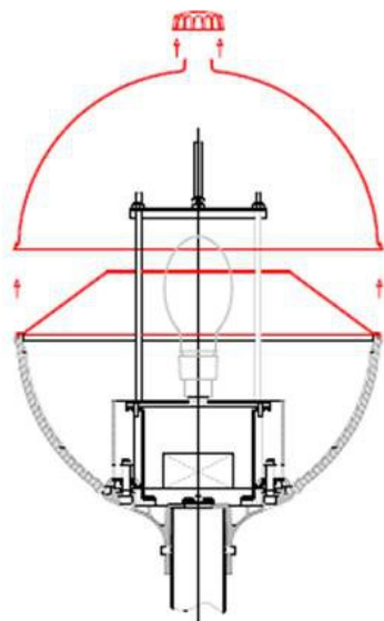
1. ABRIR LUMINARIA Y EXTRAER REFLECTOR
