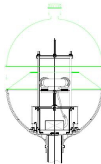
5. COLOCAR REFLECTOR Y CERRAR LUMINARIA
